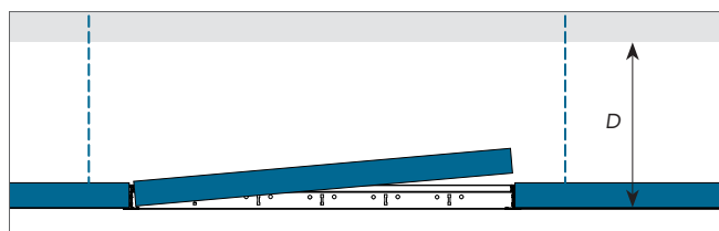
D = profondità minima di installazione.
