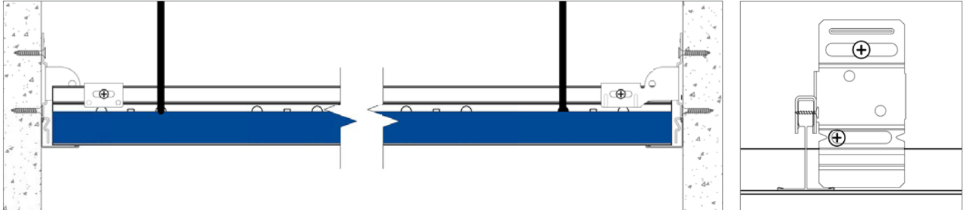
Soluzione perimetrale con pannello Rockfon bordo A.
